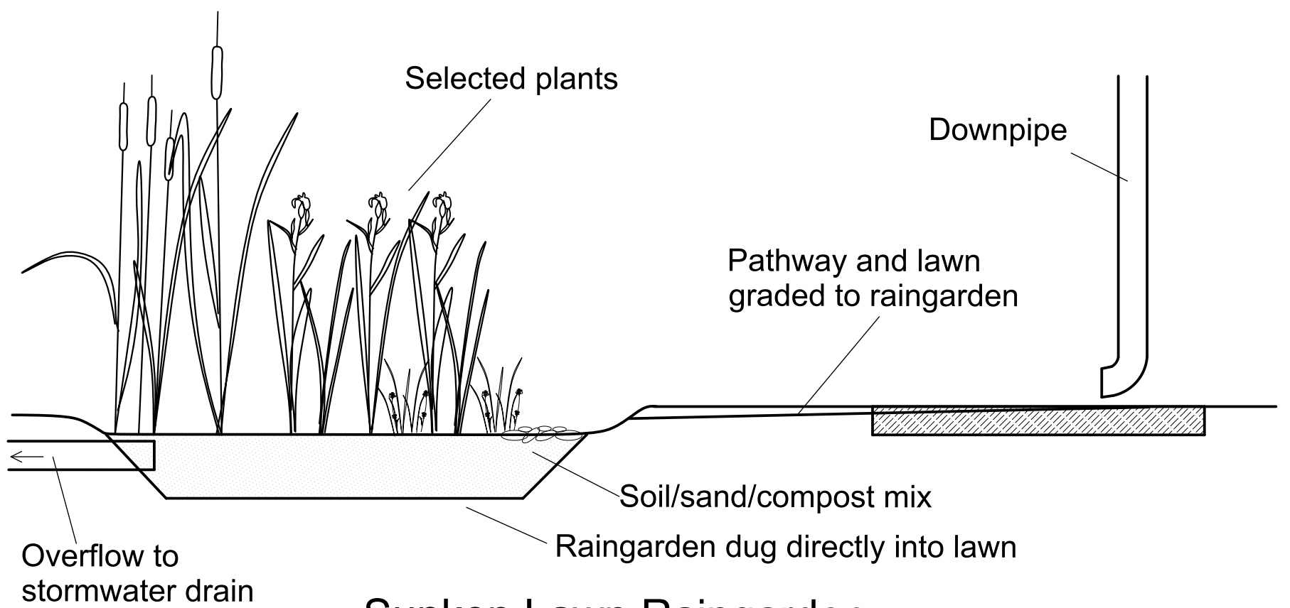
Sunken Lawn Raingarden
