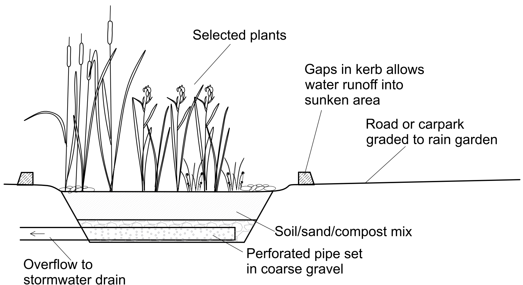
Sunken Kerbside Raingarden
